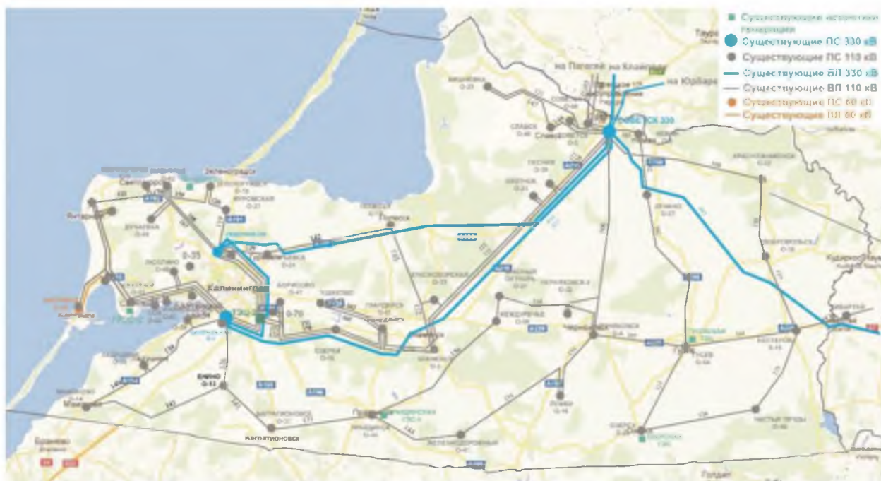
Рисунок 1. Общая карта сетей 330-110-60 кВ Калининградской области
